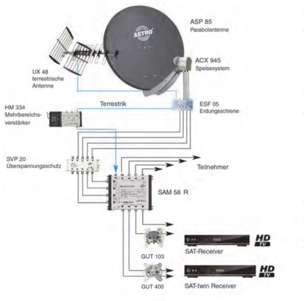
Bild 2: Anschlussbeispiel
